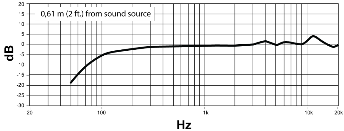
Typischer Frequenzgang
