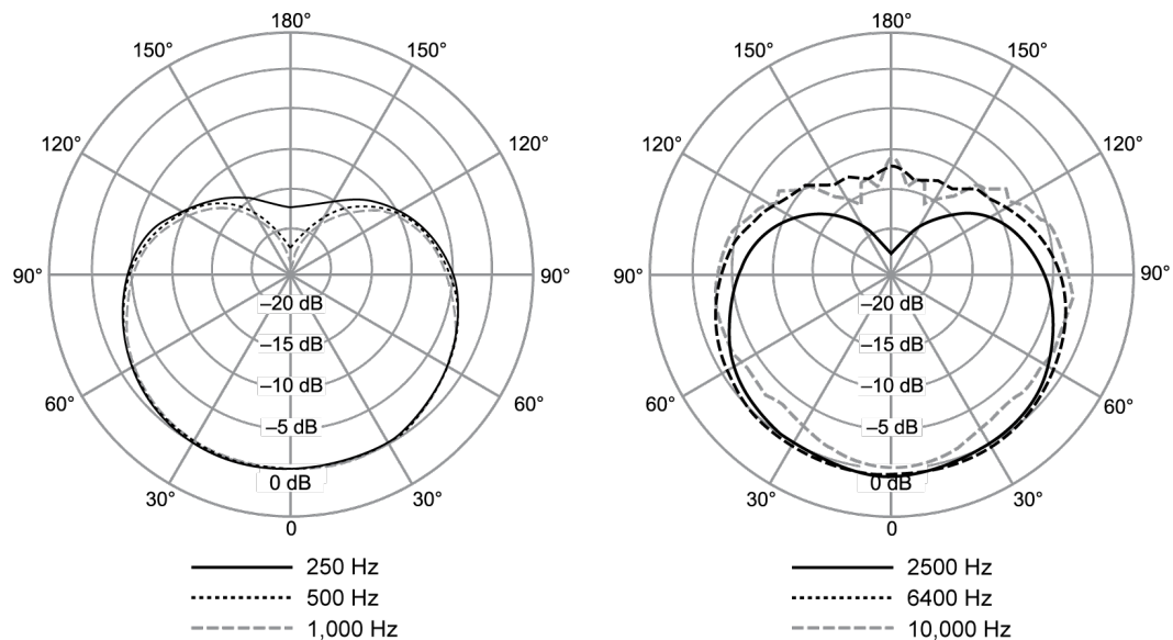
Typische Richtcharakteristik
