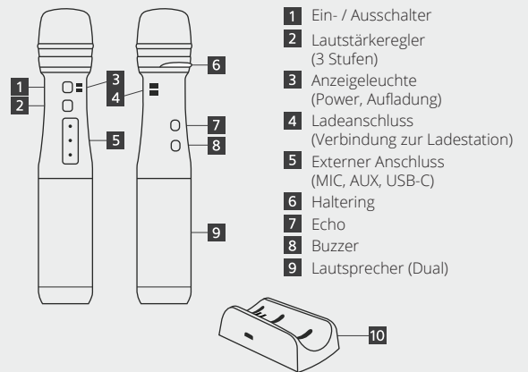
Mikrofon
