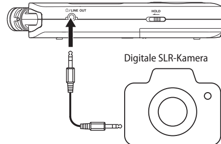
Anschluss für externes Mikrofon
