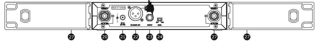
ACT-311 Einkanal-Empfänger
