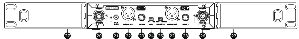
ACT-312 Zweikanal-Empfänger
