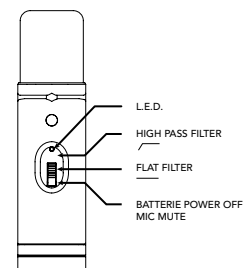
Abb. 6 – LED und Schalter
