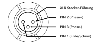
Abb. 4 – XLR-Anschluss
