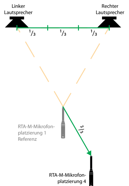
AutoEQ-Mikrofonposition 4 (optional)
